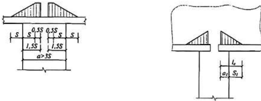
c) cũng như trên khi a > 3S d) Ở gối tựa biên của dầm liên tục và ở gối tựa của dầm đỡ một nhịp
