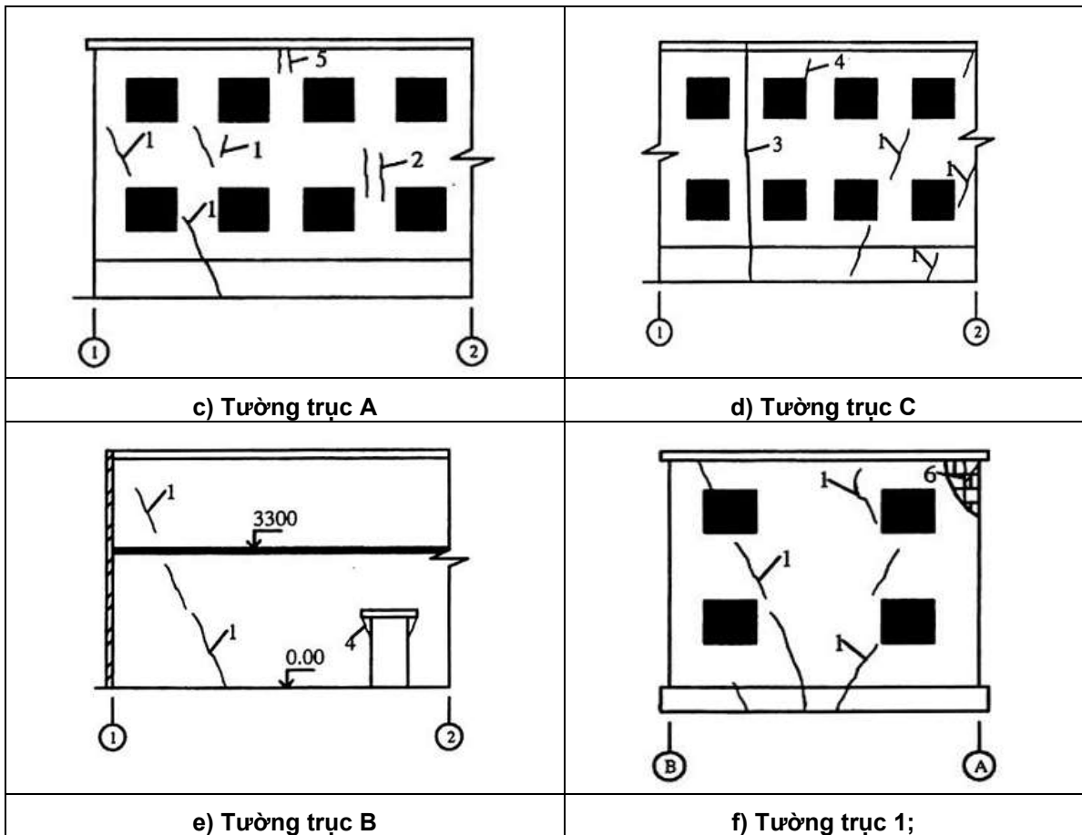
Hình C.2 - Vết nứt trong tường
