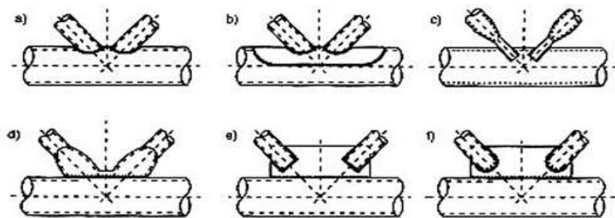
a) Liên kết hàn không bản mã; b) Liên kết hàn có bản đệm cong c,d) Liên kết hàn đầu ống đã đập bẹt; e,f) Liên kết hàn dùng bản mã
