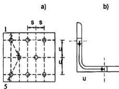
Hình 1 - Cách xác định diện tích thực
