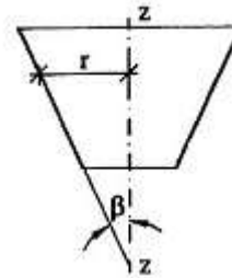
Hình 16 - Sơ đồ vỏ nón tròn xoay
