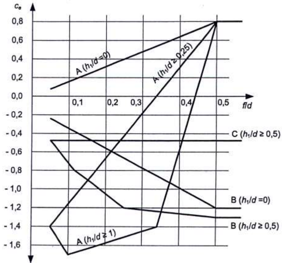
Hình F.9a - Mái chòm cầu
