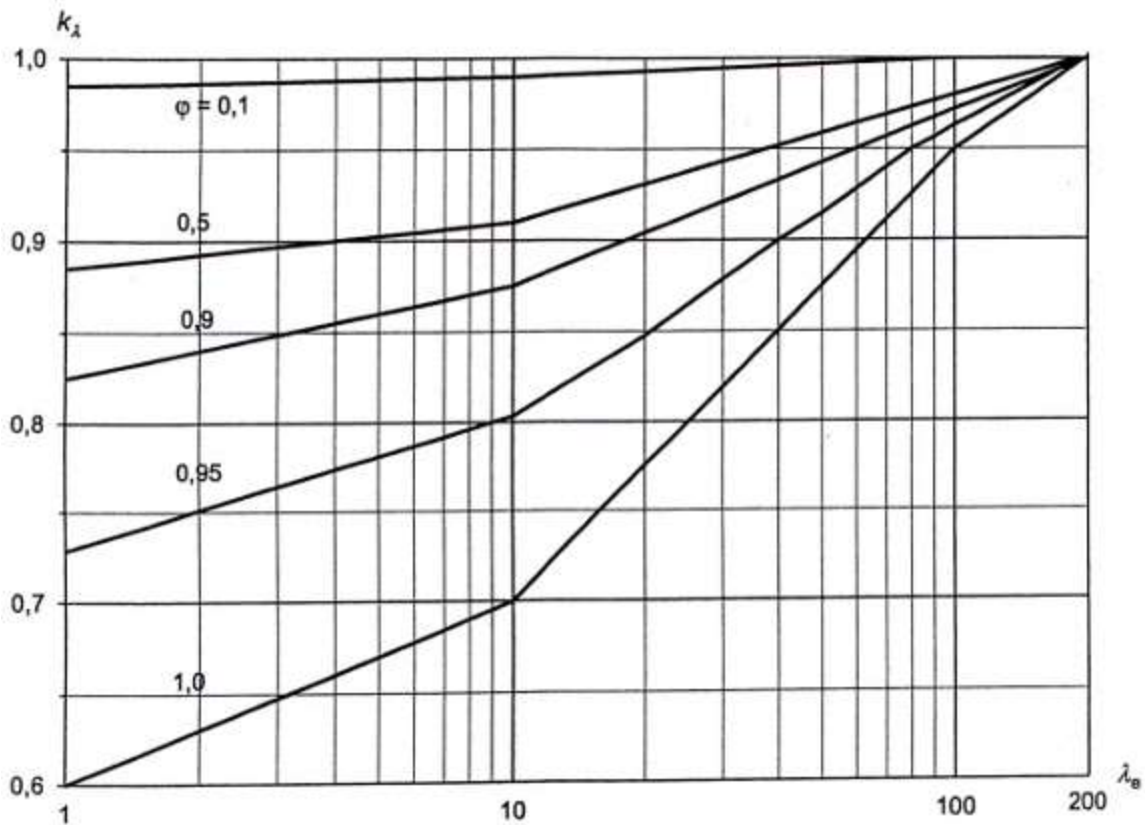
Hình F.27 - Hệ số k_\lambda
