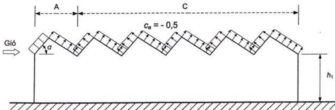
Hình F.12 - Nhà có mái răng cưa
