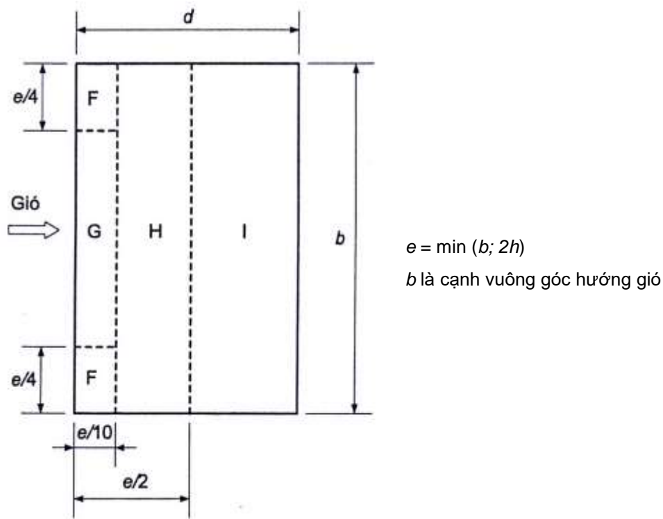
Hình F.3 - Mái bằng
