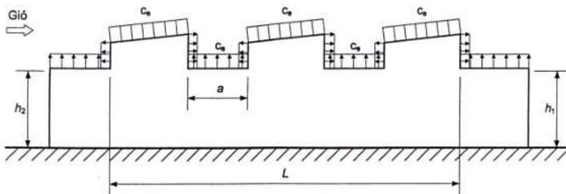
Hình F.11 - Nhà có cửa trời trên đỉnh
