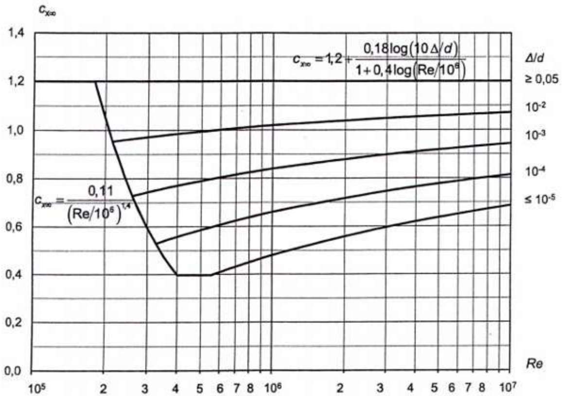
Hình F.20 - Hệ số c_{x\infty}
