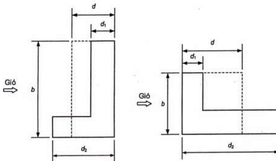
Hình E.1 - Kích thước tương đương cho một số mặt bằng phức tạp của công trình
