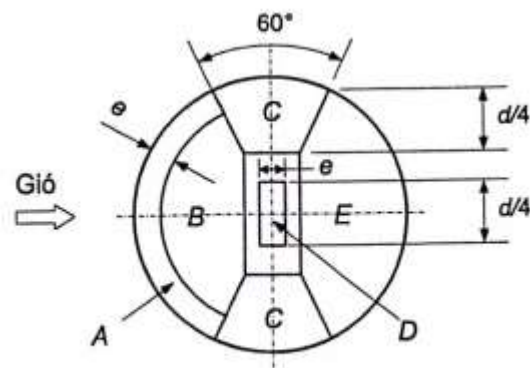
Hình F.9b - Mái nón
