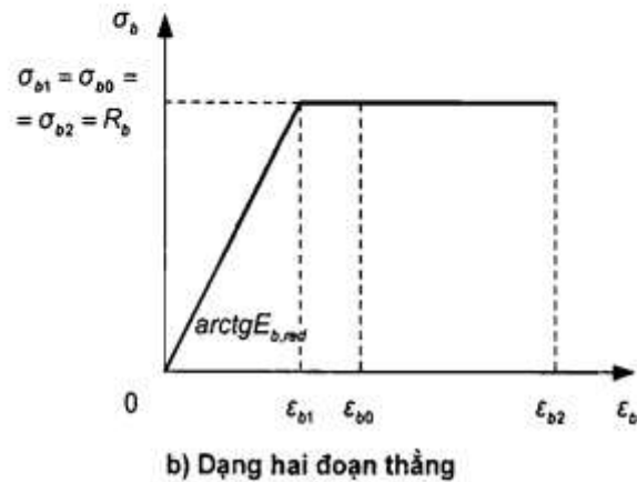
Hình 1 – Các biểu đồ biến dạng của bê tông khi nén
