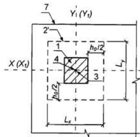
a.2) Đường bao khép kín
