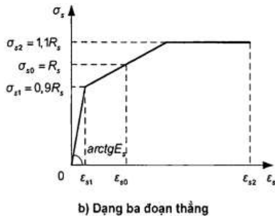
Hình 2 – Các biểu đồ biến dạng của cốt thép khi kéo
